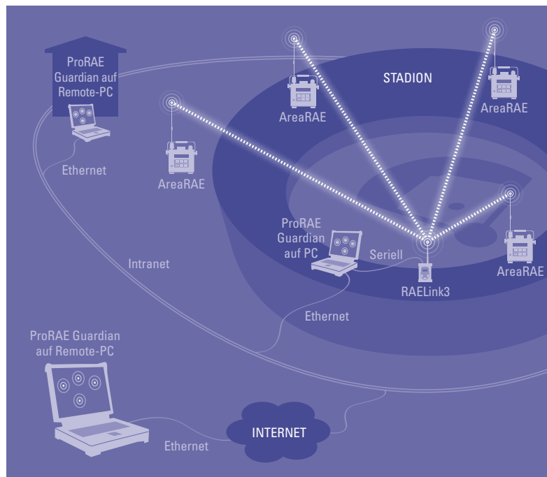
Beispiel für Einsatz des ProRAE Guardian
